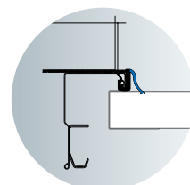
Thermische onderbreking
