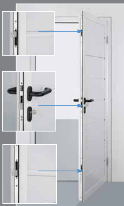
Driepuntsvergrendeling
